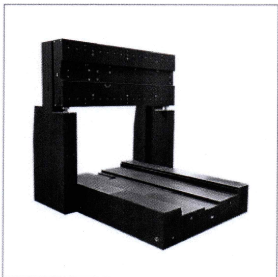
花岗石机械构件
